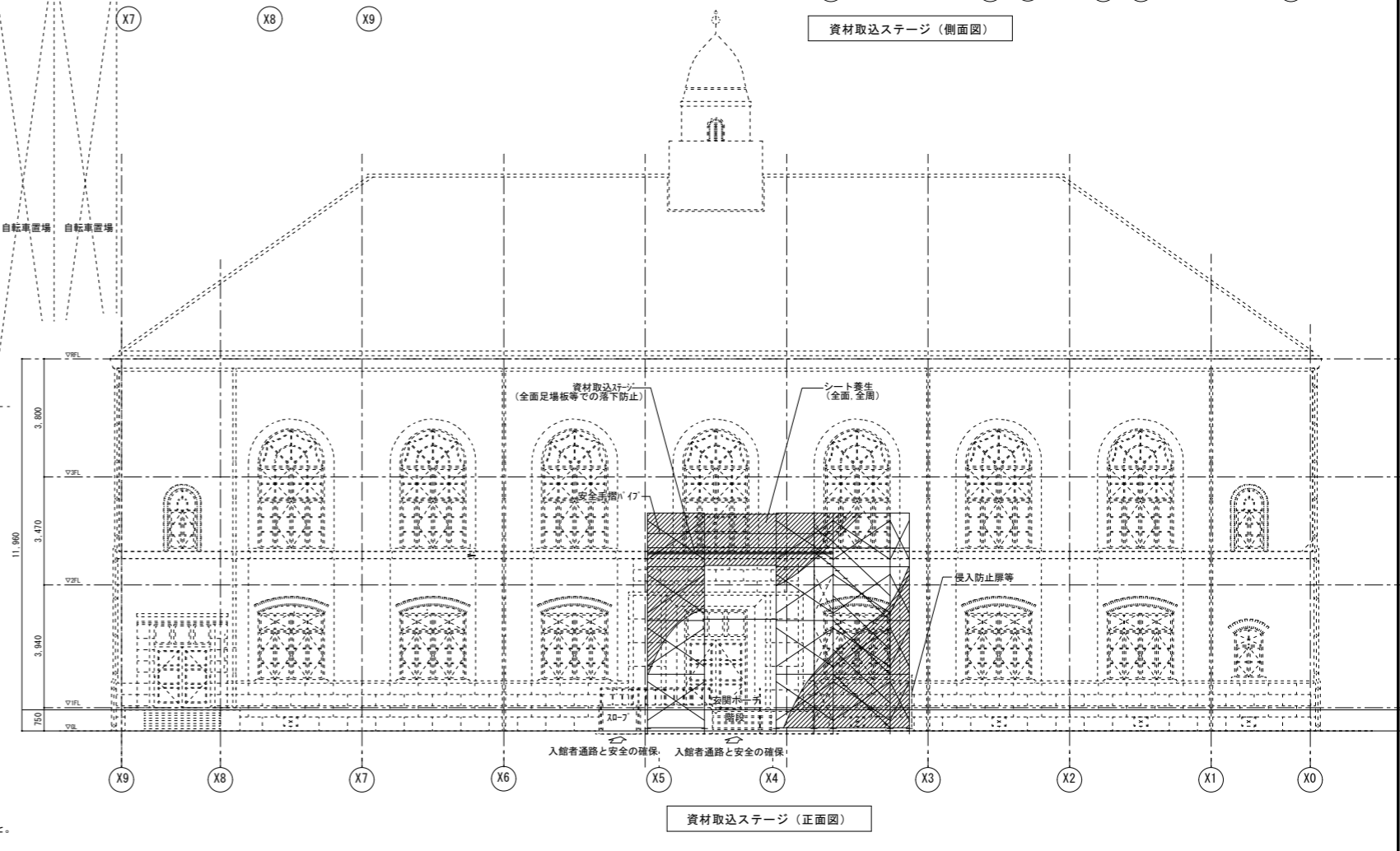
仮設計画平面図 ※誘導員を適宜配置し第三者等の事故防止を図ること。 仮設足場、資材置場、仮設間仕切等については既存部分の養生を施し損傷を与えないこと。 ※足場には安全手摺を設置するなど労働安全衛生規則等遵守のこと。 ※史料館1階は通常使用しているため、工事範囲外への防衛対策を徹底すること。
